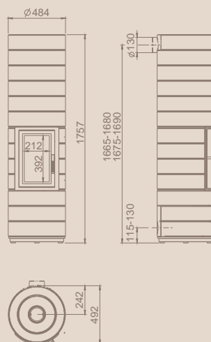
COLONA lite mit sechs Aufsatzringen
